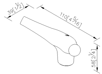
unit:mm[inch]
